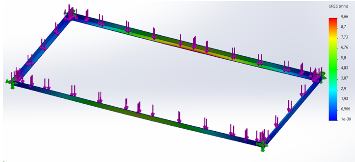
Figura 11. Zonas de desplazamientos por peso en SolidWorks
