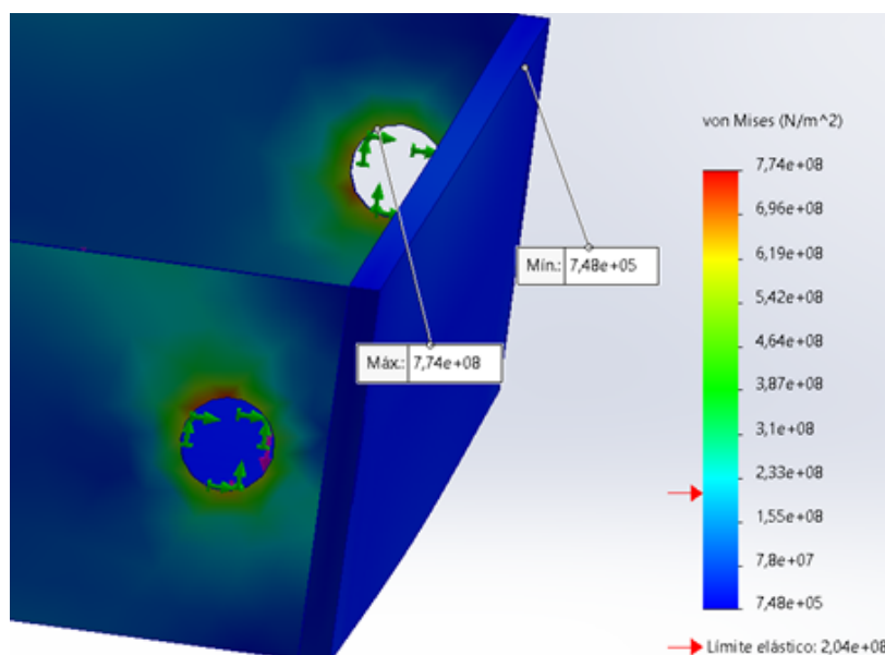
Figura 10. Áreas de tensión en ángulos en SolidWorks
