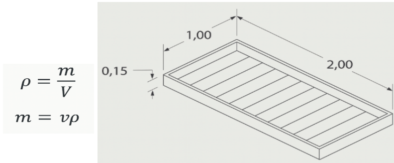
Figura 9. Dimensiones de la bandeja de cultivo
