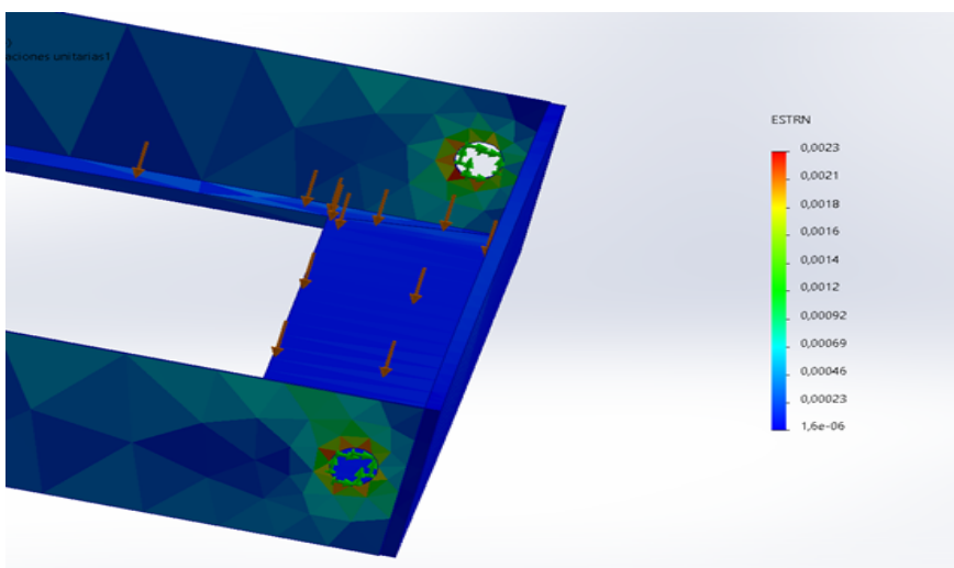
Figura 12. Deformaciones unitarias en SolidWorks
