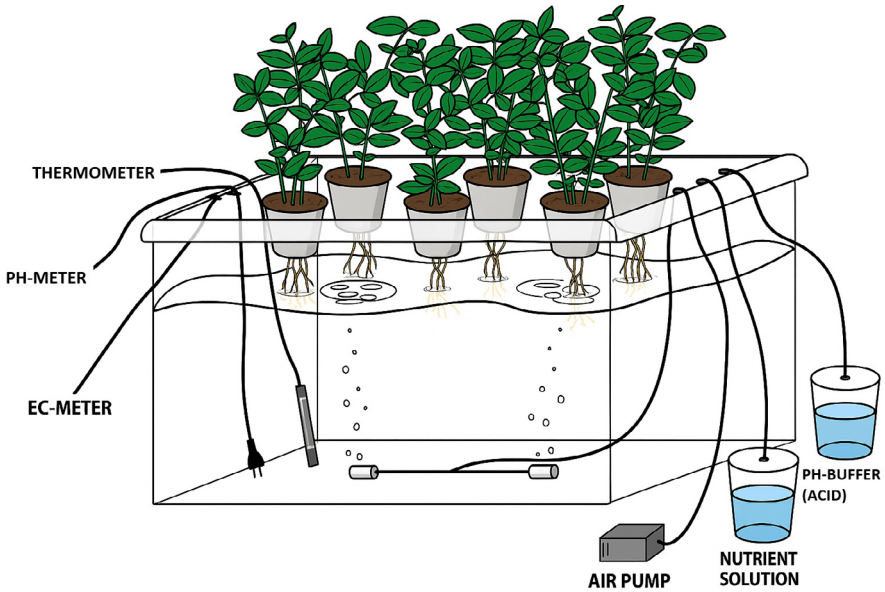
Figura 3. Balsa flotante
